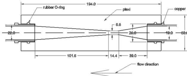
Fig. 2. Venturi orifice
