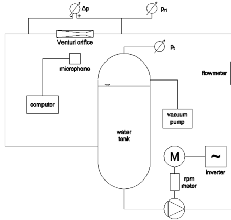
Fig. 1. Test setup
