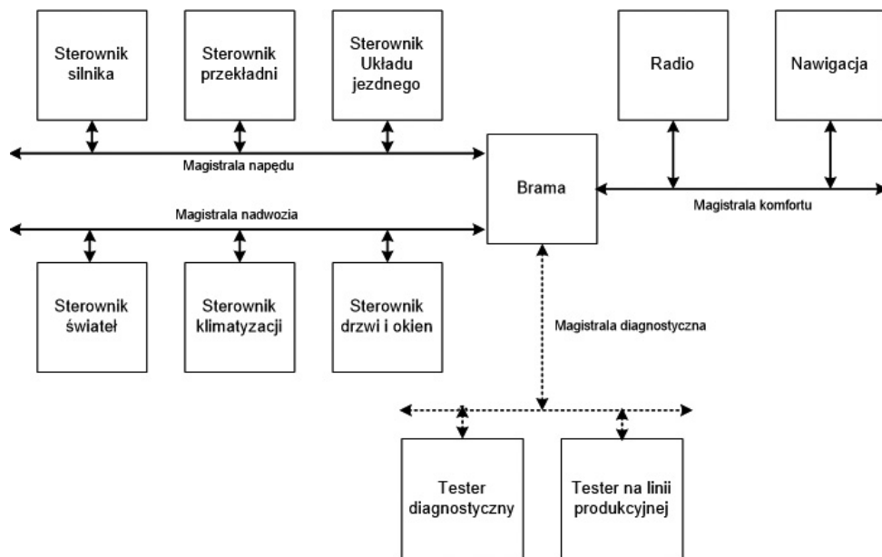
Rys. 2. System transmisji danych we współczesnym pojeździe
