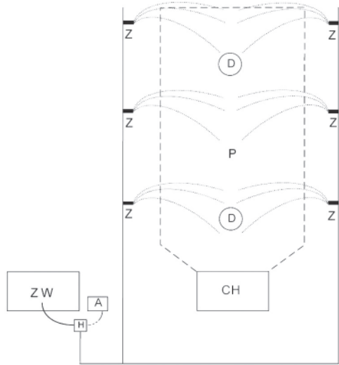
Ryc. 2. Schemat poletka podczas eksperymentów Fig. 2. Plot scheme during the experiment
