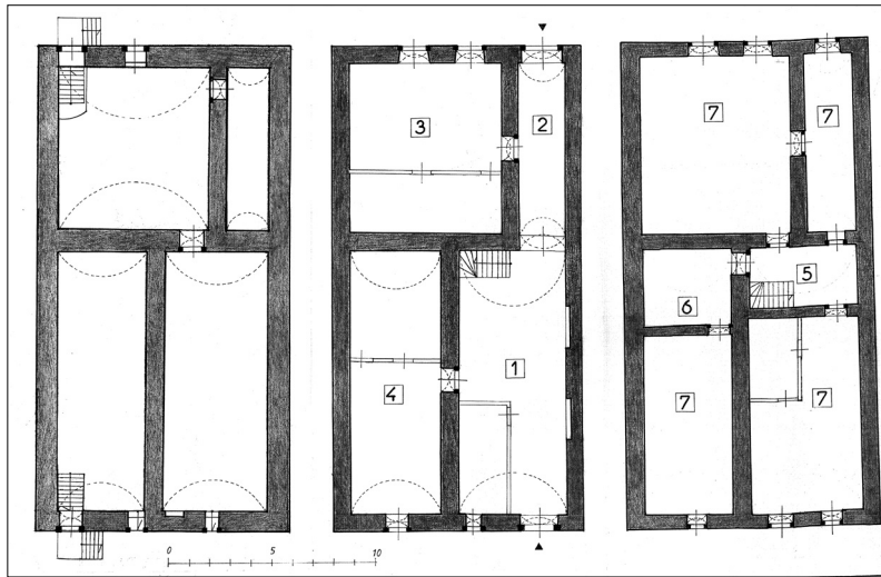
Il. 4. Rekonstrukcja budynku frontowego Starych Klas – stan z 1781 r., zapewne istniejący już w drugiej połowie XVI w. Rzuty (od lewej): piwnic, parteru i piętra. Legenda: 1 – sień w parterze; 2 – przechód w parterze; 3 – izba tylna w parterze; 4 – izba obok sieni parteru („sklep”); 5 – sień na piętrze; 6 – sionka z kuchenką na piętrze; 7 – izby na piętrze. Oprac. J. Hiżycka
