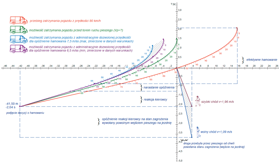
Ryc. 1. Wyniki działania programu TITAN – wykresy czasowo-przestrzenne.
