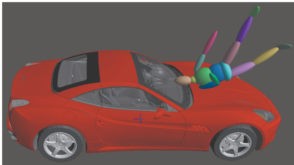
Ryc. 20. Analiza potrącenia pieszego za pomocą modelu wielobryłowego w V-SIM 5.0.
