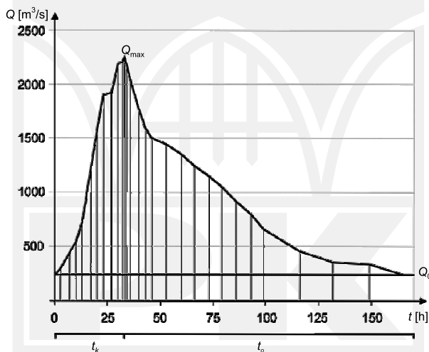
Rys. 1. Przykładowy hydrogram fali wezbraniowej dla przekroju obliczeniowego, gdzie Q_0 jest przepływem granicznym
