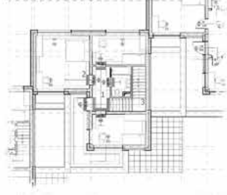
RZUT PIĘTRA SKALA 1:100
