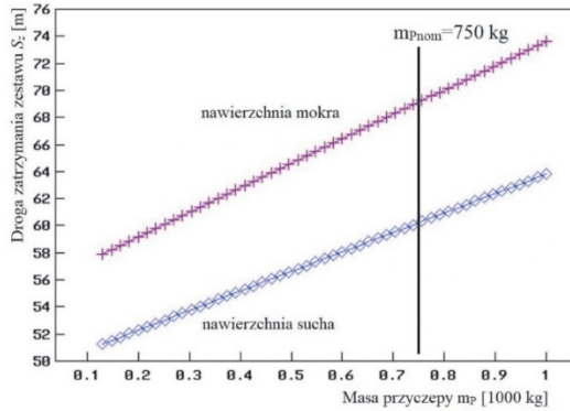
Ryc. 7. Droga zatrzymania zespołu pojazdów w funkcji masy przyczepy m_P dla analizowanych przypadków 5c i 6c.
