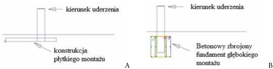
Rysunek 10. Porównanie fundamentów bollardów: płytki montaż (A), standardowy głęboki montaż (B).
