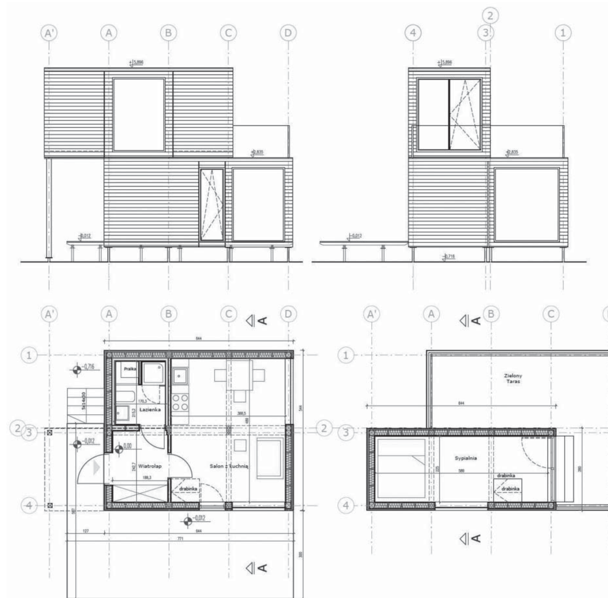
II. 2. Rysunki domu modułowego, wariant – 3 moduły w pionie, rys. M. Górka, 2018
