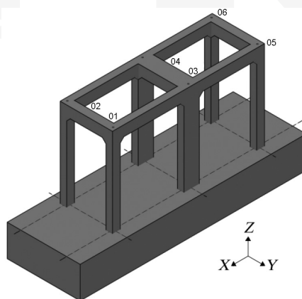
Fig. 1. Axonometric view
