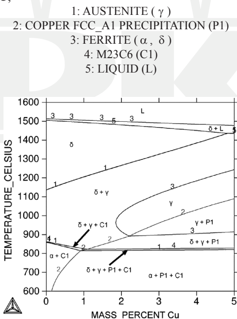
Rys. 9. Układ równowagi dla stali 410L
